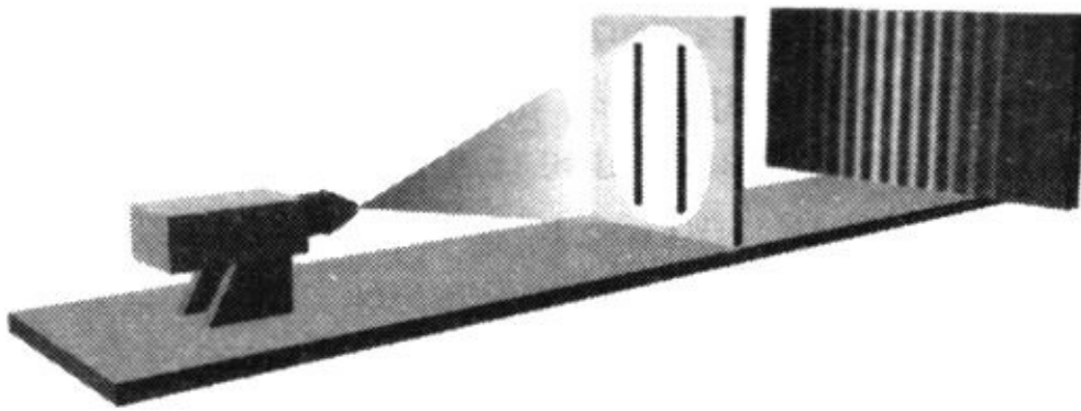
Рис. 4.8. Если свет представляет собой волну, то в тех случаях, когда открыты обе щели, будет происходить интерференция между волнами, прошедшими через разные щели
