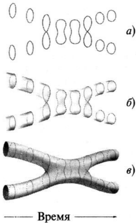
Рис. 6.7. а) Две струны, движущиеся курсом на столкновение, могут слиться и образовать третью струну, которая вслед за этим может разделиться на две струны, движущиеся по расходящимся траекториям. б) Тот же процесс, что и на рис. а), но более явно прослеживающий движение струн. в) «Замедленная киносъемка» двух взаимодействующих струн даёт мировую поверхность
