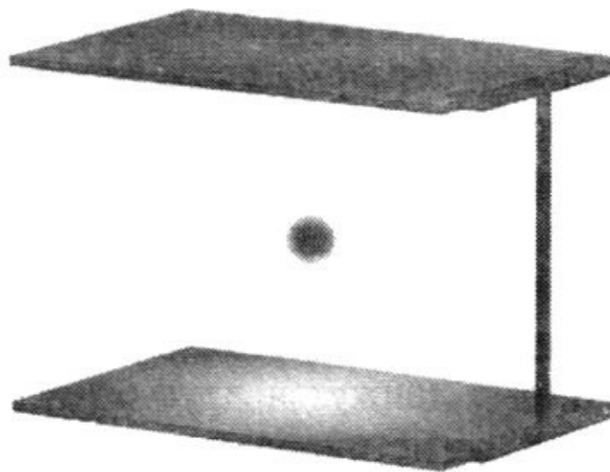
Рис. 2.1. Световые часы состоят из двух параллельных зеркал, между которыми движется фотон, поочерёдно отражаясь от каждого из них. Часы «тикают» каждый раз, когда фотон завершает свой путь туда и обратно
