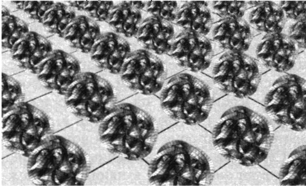
Рис. 8.10. Согласно теории струн Вселенная имеет дополнительные измерения, свёрнутые в пространство Калаби–Яу
