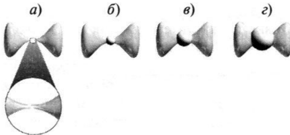
Рис. 11.4. При разрыве перетяжки пространства Калаби–Яу возникает сфера, которая сглаживает его поверхность. Исходная сфера рис. 11.3 оказывается «перестроенной»
