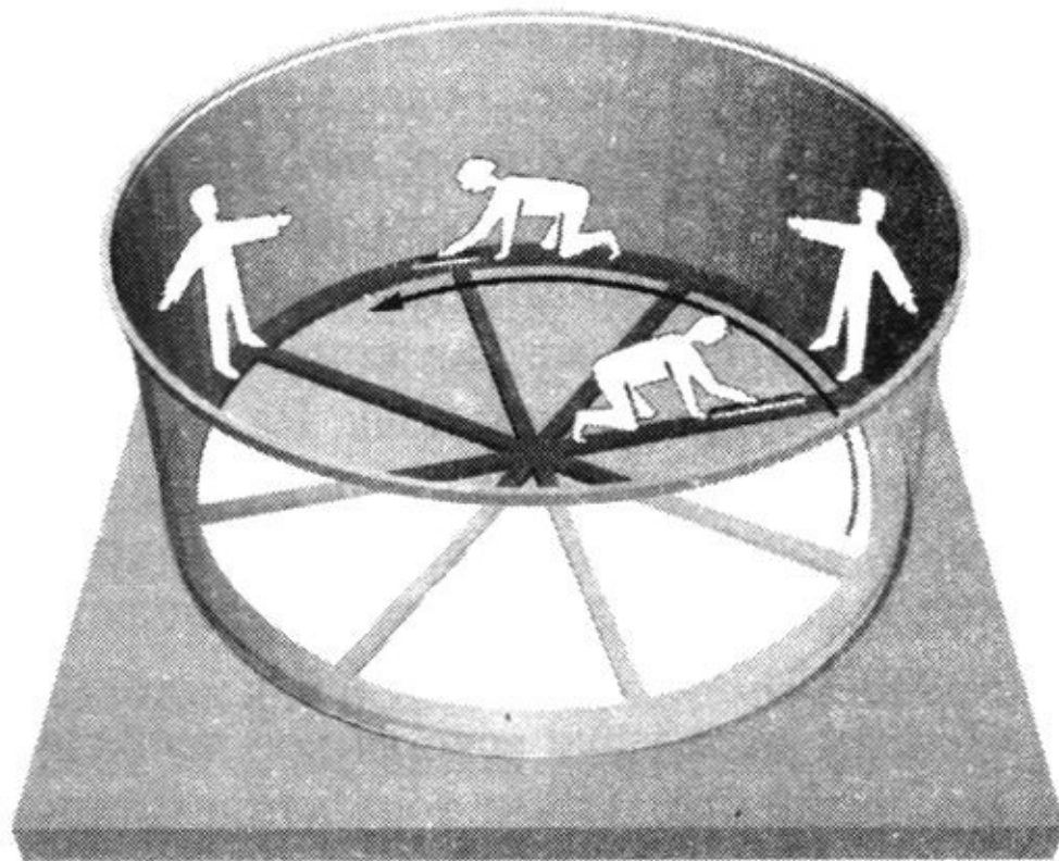
Рис. 3.1. Линейка Слима укорачивается, так как она прикладывается вдоль направления движения круга. Линейка же Джима лежит вдоль радиуса круга,
