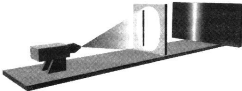
Рис. 4.5. Те же условия, как и в опыте, показанном на рис. 4.4, за исключением того, что открыта левая щель
