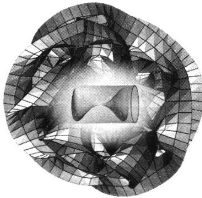
Рис. 11.6. Мировая поверхность, заматаемая струной, служит экраном, который гасит потенциально катастрофические эффекты при разрыве структуры пространства
