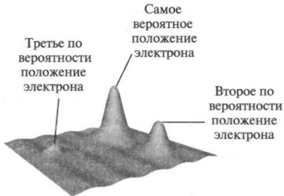
Рис. 4.9. Волна, ассоциированная с электроном, имеет наибольшую амплитуду в тех местах, где обнаружение электрона наиболее вероятно; амплитуда волны убывает по мере уменьшения вероятности обнаружения электрона
