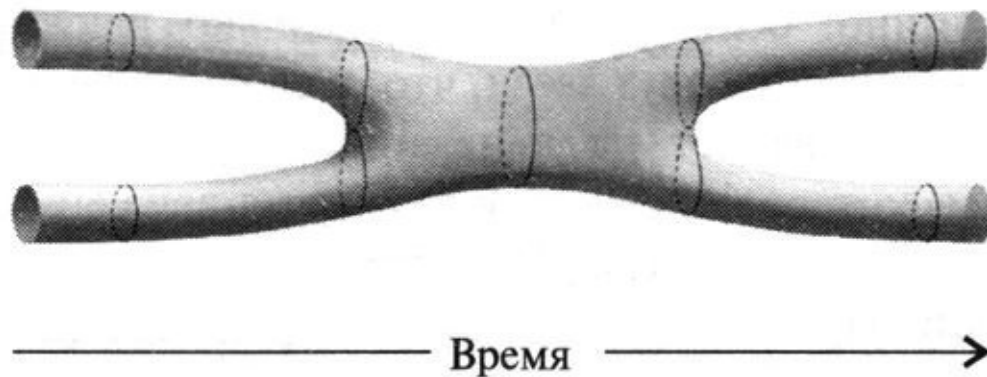
Рис. 12.3. Струны взаимодействуют, соединяясь и разделяясь
