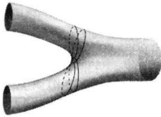
Рис. 6.10. Мнения Джорджа и Грейс по вопросу о месте, в котором произошло взаимодействие, разойдутся
