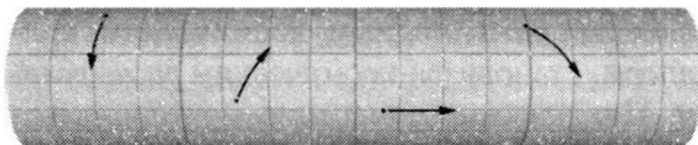
Рис. 10.2. Точечные частицы, движущиеся по цилиндру
