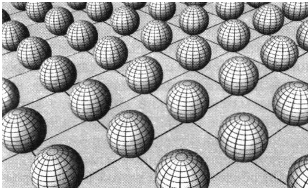
Рис. 8.7. Два дополнительных измерения, свёрнутые в сферу
