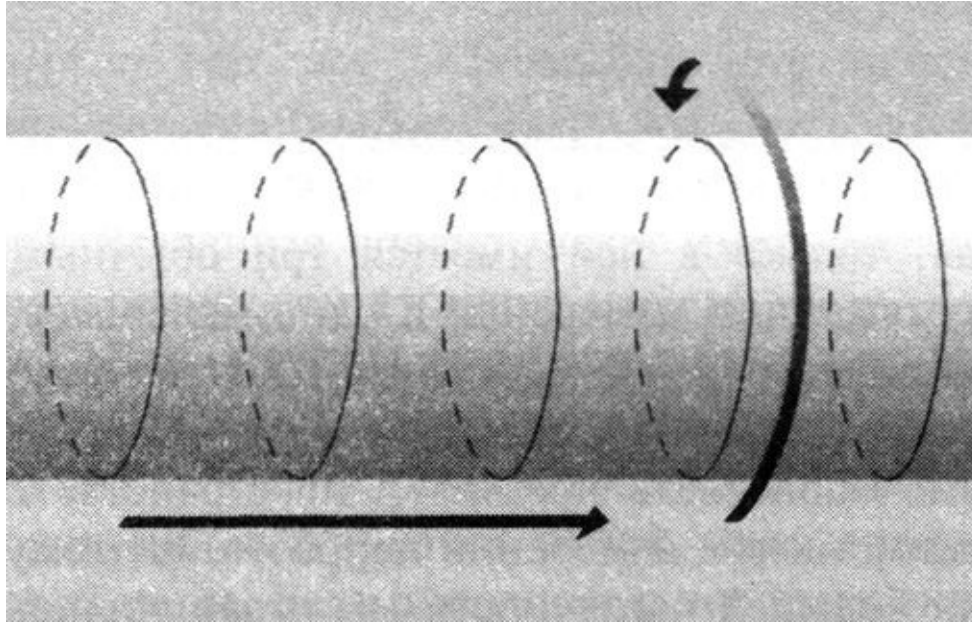
Рис. 8.2. Поверхность Садового шланга является двумерной. Одно измерение (идущее вдоль горизонтальной оси шланга), отмеченное прямой стрелкой, является длинным и протяжённым. Другое измерение (окружность шланга), отмеченное круговой стрелкой, является маленьким и свёрнутым
