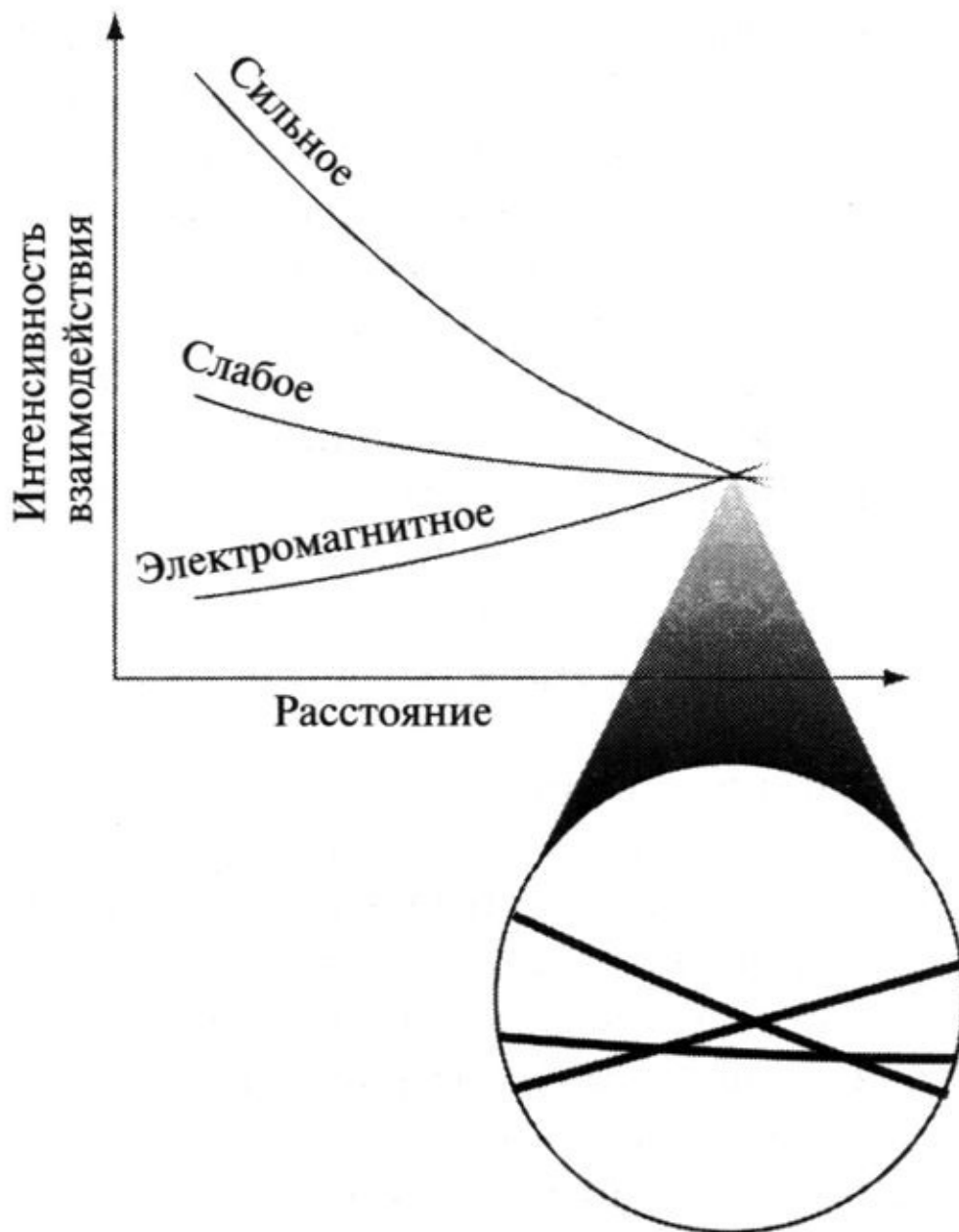
Рис. 7.2. Уточнение расчёта интенсивностей взаимодействий показало, что без
