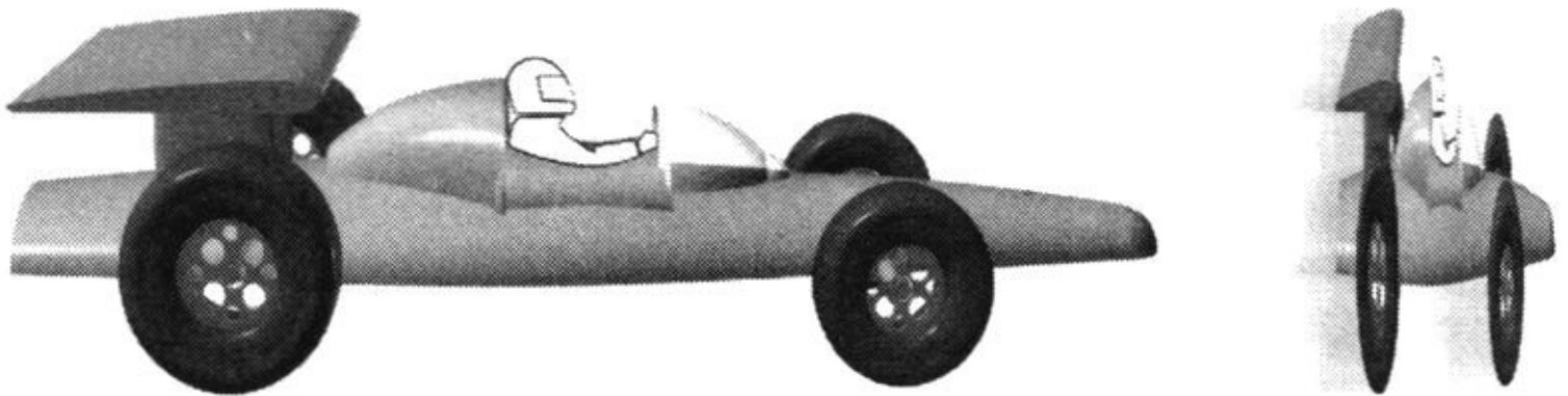
Рис. 2.4. Движущийся объект сокращается в направлении своего движения
