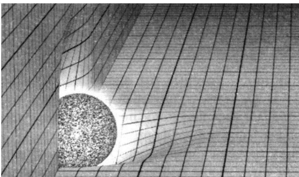
Рис. 3.6. Пример искривлённого трёхмерного пространства, окружающего Солнце
