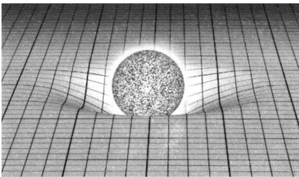
Рис. 3.4. Массивное тело, такое как Солнце, заставляет структуру пространства искривляться подобно тому, как деформируется резиновая плёнка, если на неё положить шар для боулинга
