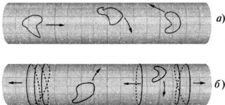
Рис. 10.3. Струны на цилиндре могут двигаться в двух конфигурациях — «ненамотанной» или «намотанной»
