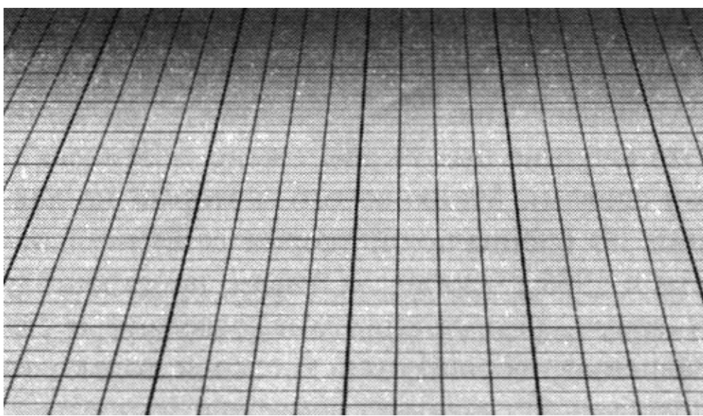
Рис. 3.3. Схематическое представление плоского пространства
