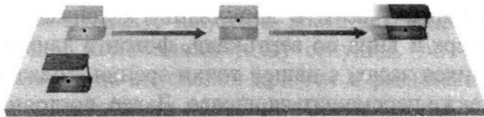
Рис. 2.2. На переднем плане расположены неподвижные световые часы. Световые часы, расположенные в глубине, движутся с постоянной скоростью
