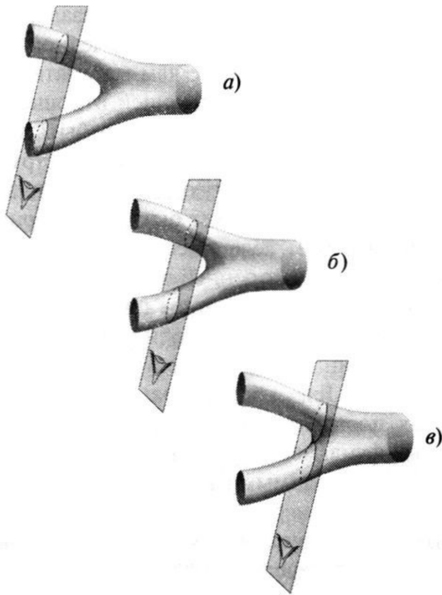
Рис. 6.9. Две исходные струны (с точки зрения Грейс) в три последовательных момента времени. В моменты а) и б) струны сближаются, в момент в) , с её точки зрения, они впервые соприкоснулись
