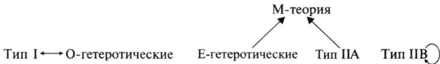
Рис. 12.9. Стрелки обозначают отношения дуальности для теорий
