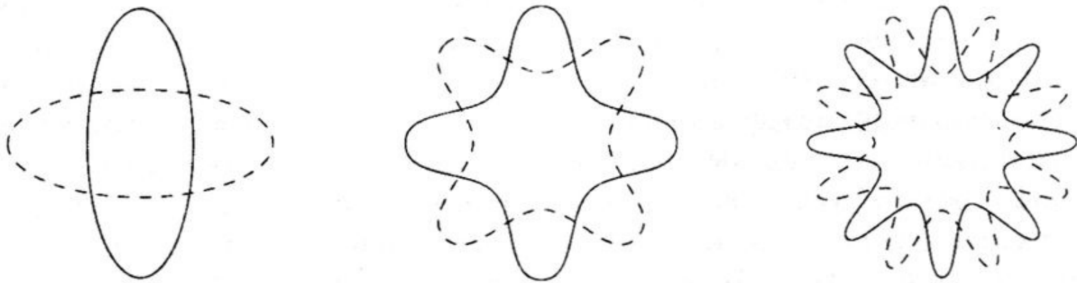
Рис. 6.2. Петли теории струн имеют резонансные моды колебаний, похожие на моды резонансных колебаний скрипичных струн. При этом вдоль длины струны укладывается в точности целое число максимумов и минимумов
