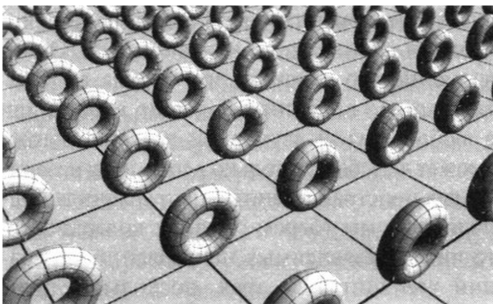
Рис. 8.8. Два дополнительных измерения, свёрнутые в баранку (тор)
