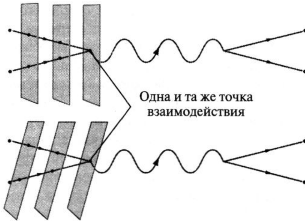
Рис. 6.11. Наблюдатели, находящиеся в относительном движении, придут к согласию о месте и времени взаимодействия между двумя частицами
