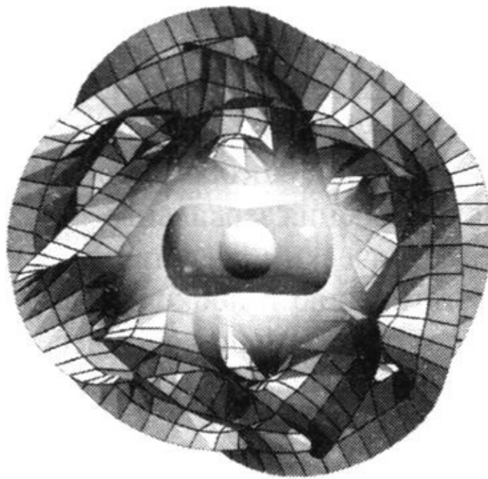
Рис. 11.2. В выделенной области внутри пространства Калаби–Яу находится сфера
