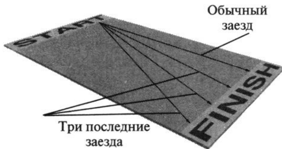
Рис. 2.5. Из-за того что Солнце в конце дня слепило в глаза, в течение последних трёх заездов Слим двигался под всё более увеличивающимся углом
