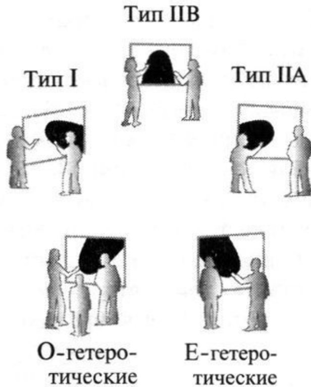
Рис. 12.1. Многие годы физики, работавшие с пятью теориями струн, думали, что они исследуют совершенно различные теории
