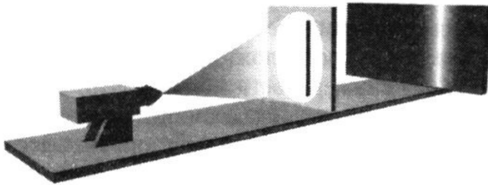
Рис. 4.4. В этом опыте открыта правая щель, в результате изображение на фотопластинке будет выглядеть, как показано на рисунке
