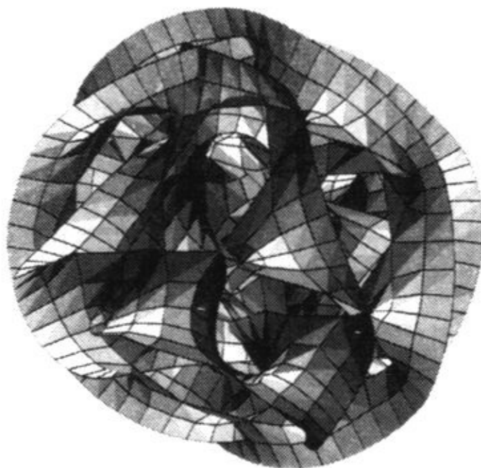
Рис. 8.9. Пример пространства Калаби–Яу
