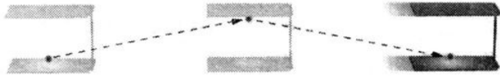
Рис. 2.3. С нашей точки зрения фотон в движущихся часах перемещается по диагональному пути
