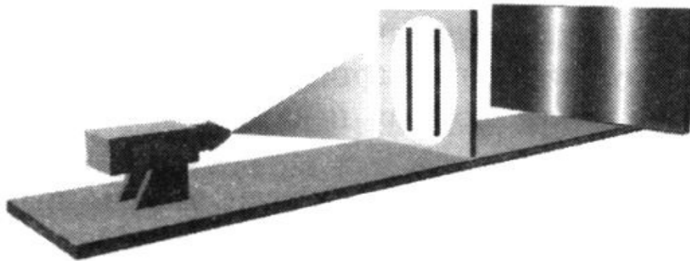
Рис. 4.6. Ньютоновская корпускулярная модель предсказывает, что когда будут открыты обе щели, картина на фотопластинке будет представлять собой объединение картин, показанных на рис. 4.4 и 4.5
